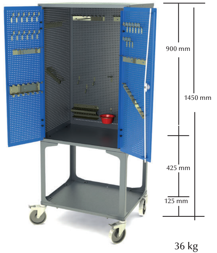
VERKTYGSVAGN MED HÅLLARE OCH SYMBOLER FÖR 105 VERKTYG TOOL TROLLEY WITH SYMBOLS AND HOLDER FOR 105 TOOLS Article no. 900105
